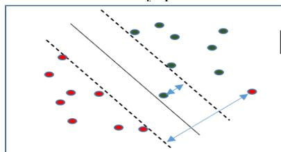
شکل ۲. خط جداکننده بردار پشتیبان با حاشیه‌های نرم
