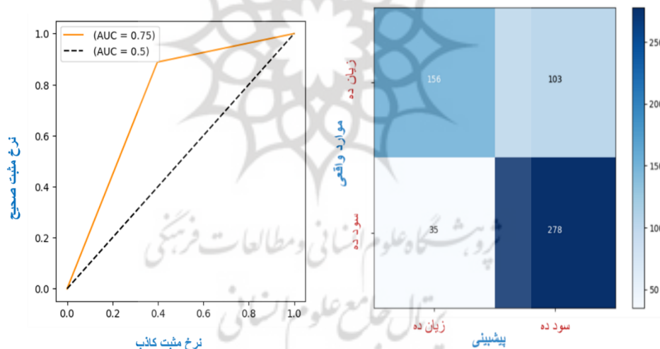
شکل ۳. ماتریس اغتشاش و منحنی ROC الگوریتم درخت تصمیم
