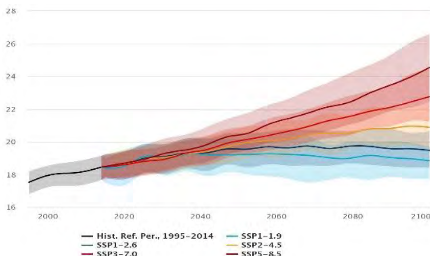
شکل ۳- پیشبینی میانگین دما بر اساس سناریوهای SSP توسط IPCC در مورد ایران منبع: CCKP (۱۱)
