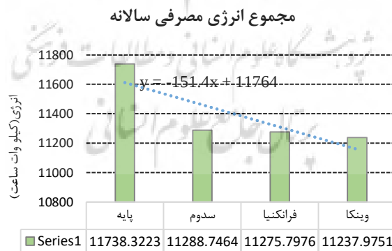
شکل ۵: مجموع انرژی مصرفی سالانه در مدل‌های ساختمانی
