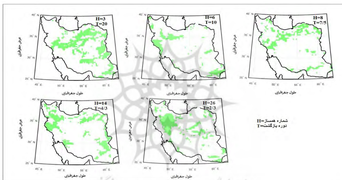
شکل ۶. توزیع مکانی چرخه‌های معنادار همسازهای ۳، ۶، ۸، ۱۴، ۲۶ بارش طی دوره آماری ۱۹۶۳-۲۰۲۲
