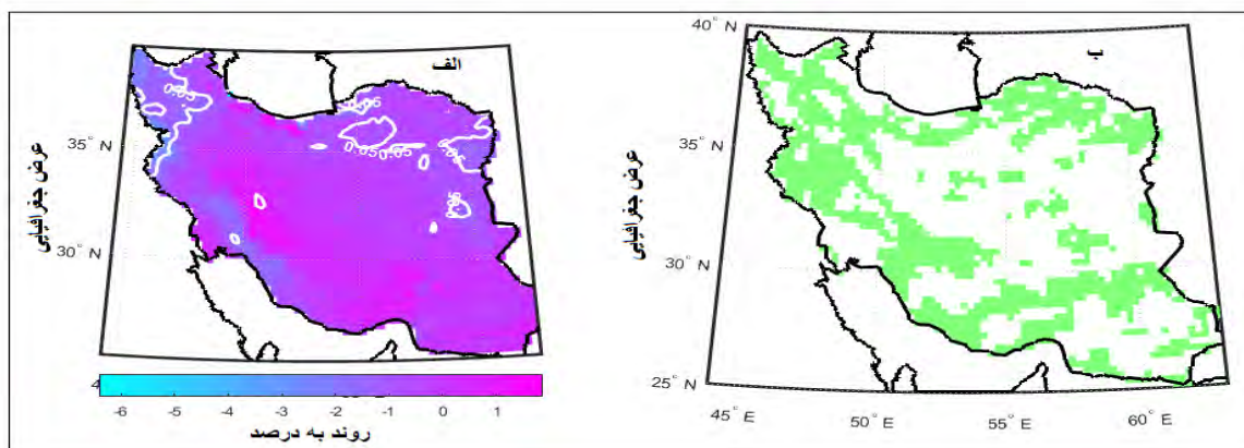
شکل ۲. توزیع مکانی روند بارش (الف) و چرخه‌های معنادار همساز اول بارش سالانه طی دوره آماری ۱۹۶۳-۲۰۲۲
