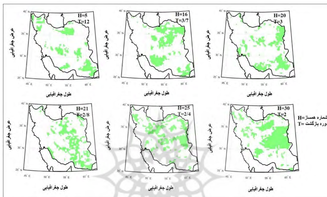
شکل ۵. توزیع مکانی چرخه‌های معنادار همسازهای ۵، ۱۶، ۲۰، ۲۱، ۲۵، ۳۰ بارش طی دوره آماری ۱۹۶۳-۲۰۲۲
