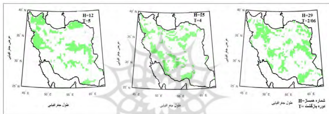
شکل ۳. توزیع مکانی چرخه‌های معنادار همسازهای ۱۲، ۱۵ و ۲۹ بارش طی دوره آماری ۱۹۶۳-۲۰۲۲
