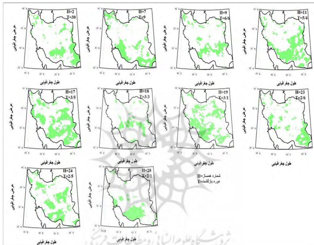
شکل ۴. توزیع مکانی چرخه‌های معنادار همسازهای ۲، ۷، ۱۱، ۱۷، ۱۸، ۱۹، ۲۳، ۲۴، ۲۸ بارش طی دوره آماری ۲۰۲۲-۱۹۶۳
